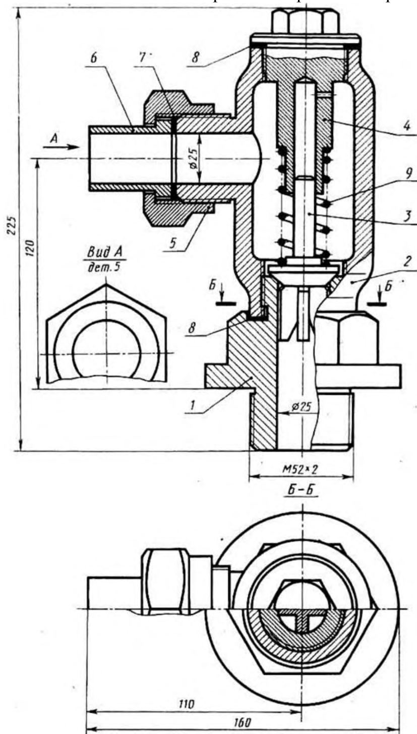
Рис. 44. Клапан обратный
