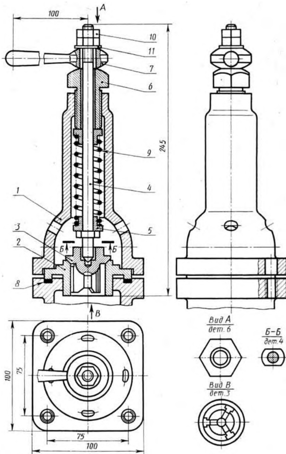
Рис. 42. Клапан предохранительный
