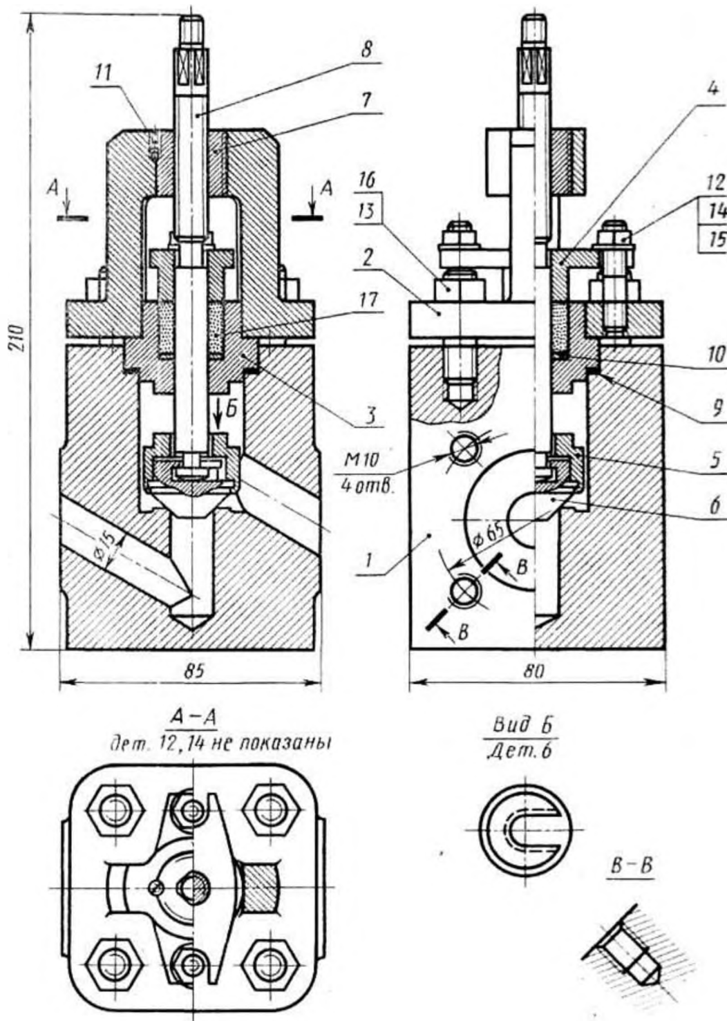
Рис. 43. Вентиль шаровый
