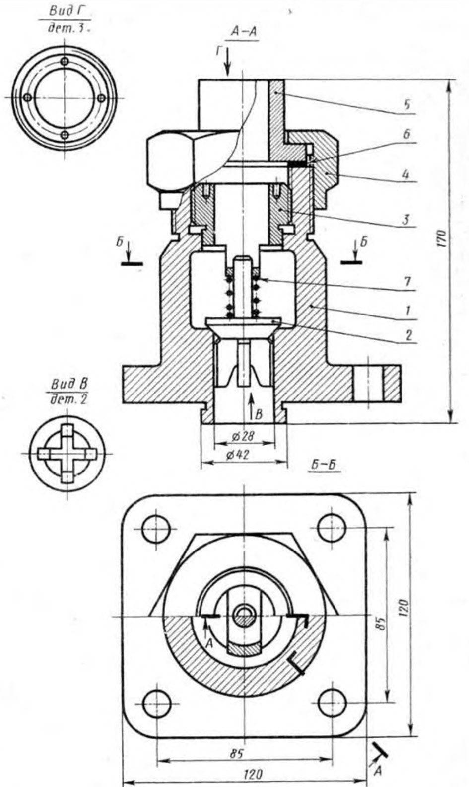
Рис. 41. Клапан обратный
