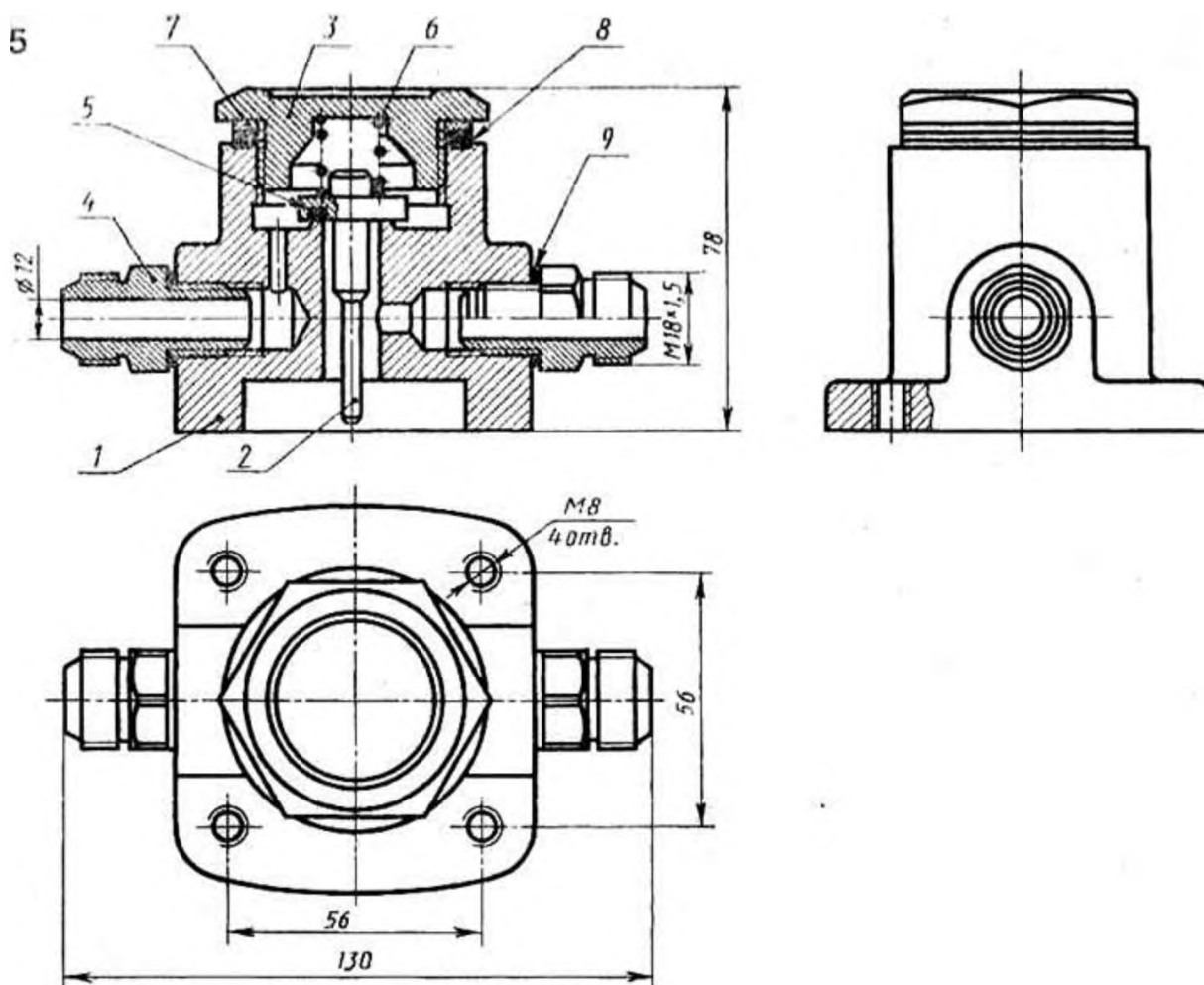
Рис. 45. Клапан предохранительный
